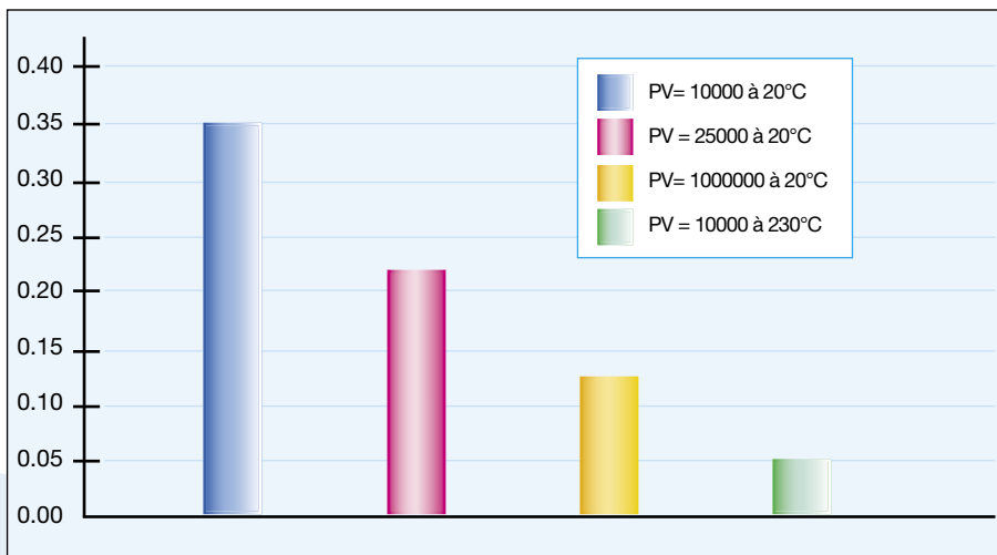
Évolution du coefficient de friction du MELDIN 7021 pour des conditions de valeurs PV différentes
